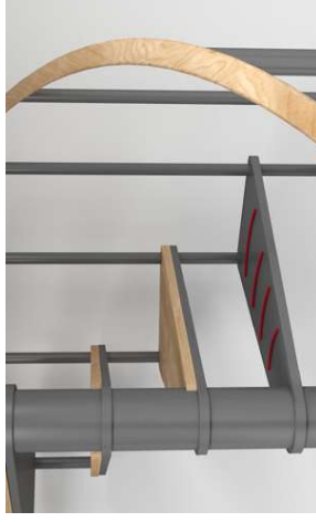
Klebung im Treppenaufbau
